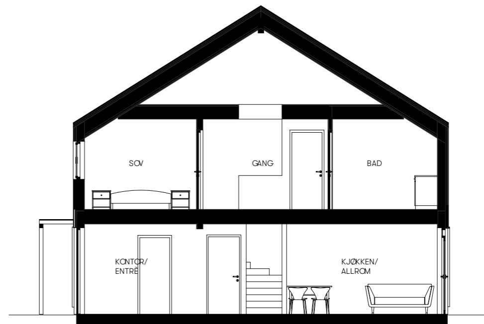
SNITT 1:100
